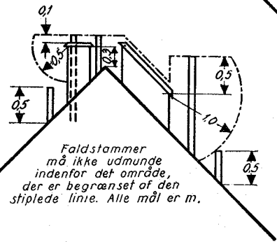
Fig. 45: Eksempel på installation med udluftede sideledninger. Sideledningernes tilslutning til ventilationsledningen skal ske over gulv, herfra dog undtaget nederste sideledning. Faldstammen kan ikke udluftes gennem sideledningen i øverste etage. Fig. 46-47: Anbringelse af faldstammers udluftning over tag i forhold til tudtagsten og hætter for rumaftræk.
