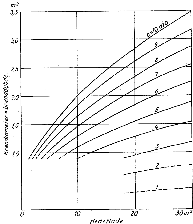
Fig. 68: Diagram for dimensionering af udblæsningsbrønde for dampkedler med hedeflade indtil 30 \text{ m}^2 . Mindste brøndstørrelse: diam. 1,0 \text{ m} , dybde 1,0 \text{ m} .
