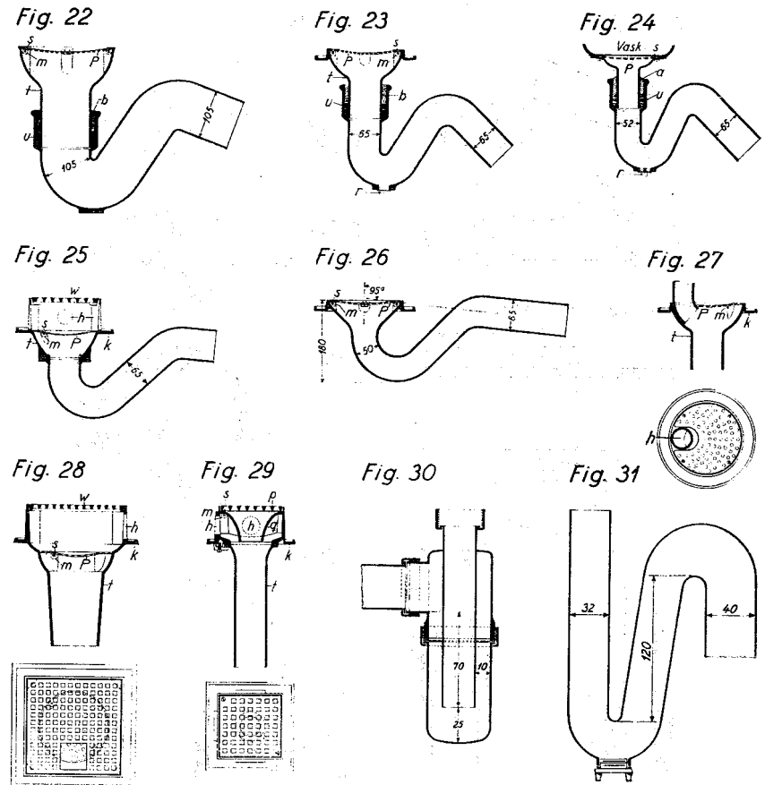
Fig. 22-24: Almindelige støbejernsvandlås med afløbstragt. Fig. 25: „Saxofon- vandlås“ af støbejern med firkantet afløbsskål. Fig. 26: „Saxofonvandlås“ af stø- bejern med lav afløbstragt. Fig. 27: Almindelig støbejernstragt med udskæring i messingristen for afløb fra håndvask eller badekar. Fig. 28: Afløbstragt med fir- kantet afløbsskål med fastskruet messingrist og løs overrist af støbejern. Fig. 29: Afløbstragt med firkantet afløbsskål med fastskruet støbejernsrist og underlig- gende tragt for at hindre vand fra sidetilløbene i at stemme op gennem risten. Fig. 30: Pungvandlås af forkromet messing. Fig. 31: Uudsugelig 32/40 mm bly- vandlås.
