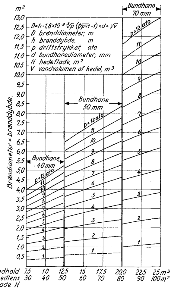
Fig. 69: Diagram for dimensionering af udblæsningsbrønde for dampkedler med hedeflade 30-100 \text{ m}^2 . Mindste brøndstørrelse: diam. 1,0 \text{ m} , dybde 1,0 \text{ m} . Såfremt kedlens bundhane ikke har den i diagrammet forudsatte størrelse, skal den fundne brøddimension multipliceres med forholdet mellem den virkelige diameter af bundhansen og den i diagrammet forudsatte.
